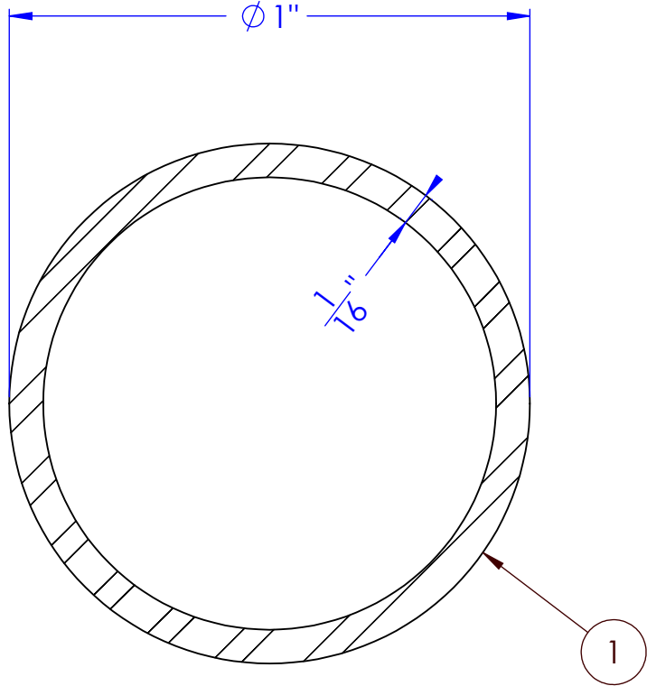
SECTION C-C ESCALE 3 : 1
